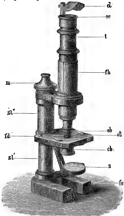
Фиг. 2. Штативъ VII a Цейсса съ рисовальною призмою cl \frac{1}{2} , наст. вел. fs ножка, sl'' нижний, sl'' верхняя часть столбика, ot предметный столикъ, cb цилиндрическія діафрагмы, fd нажимы, s зеркало, m микрометрической винтъ, fh гильза, t трубка, ob объективъ, oc окуляръ.
